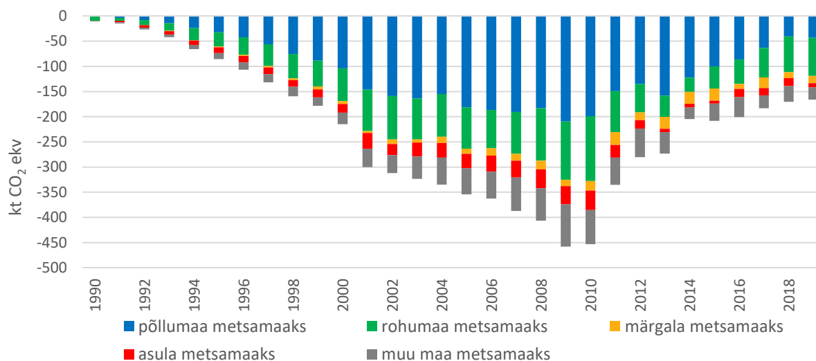
Joonis 2.16 Metsastunud ala KHG aastane netosidumine varasema maakatgoria järgi (LULUCFi määratlus)
