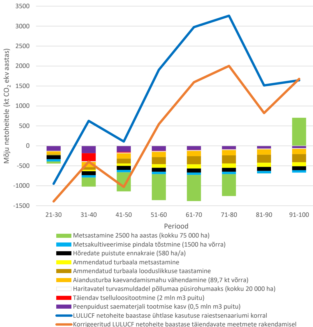
Joonis 7.2 LULUCFi täiendavate meetmete koondstsenaariumi mõju sektori netoheittele 2021.–2100. aastal (baasstsenaarium on ühtlase kasutuse raiestsenaarium)
